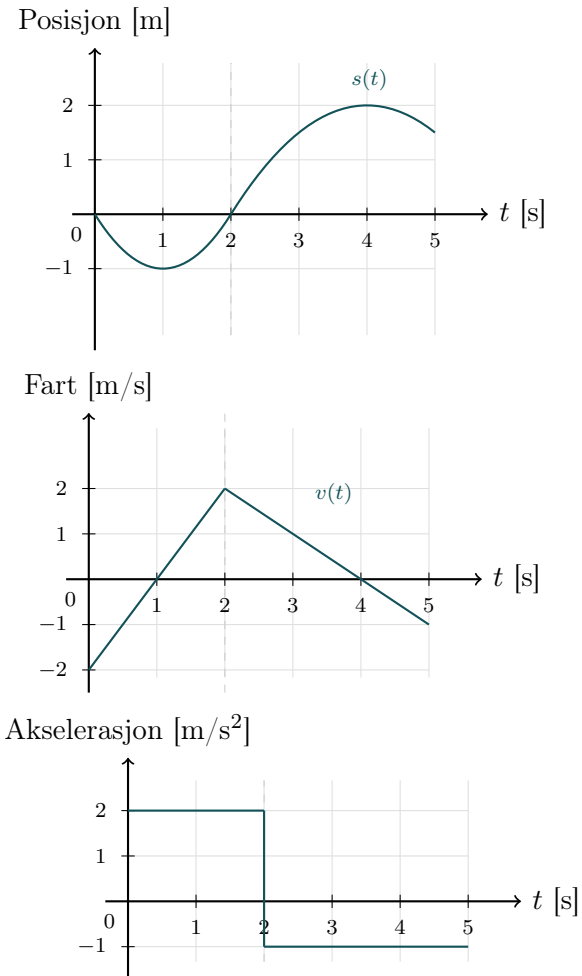
Figur 3.4: Posisjon, fart og akselerasjon ved varierende akselerasjon ( s_0 = 0 , v_0 = -2 \text{ m/s} ; a_1 = 2 \text{ m/s}^2 for t \in [0, 2 \text{ s}] og a_2 = -1 \text{ m/s}^2 for t \in [2, 5 \text{ s}] ).
