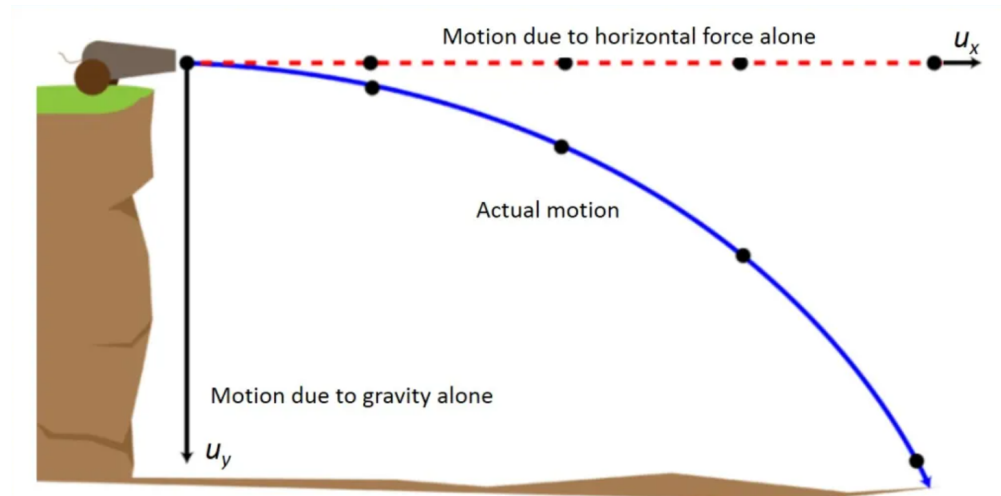
Figur 3.5: Prosjektilbevegelse
